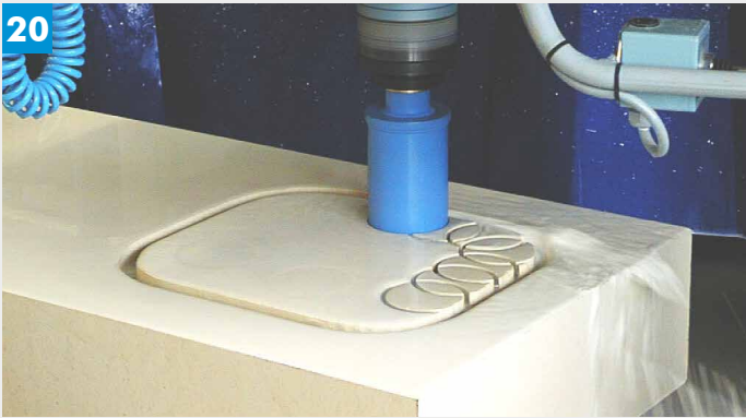
EN Core drilling in massive limestone FR Perçage évier dans la masse DE Kernbohrungen im massiven Sandstein ES Taladro de fregadero macizo
