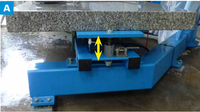
EN Granite tilting work table (0 to 1°) FR Table de travail inclinable en granit (0 à 1°) DE Neigbarer Arbeitstisch aus Granit (0 bis 1°) ES Mesa de trabajo inclinable de granito (0 a 1°)
