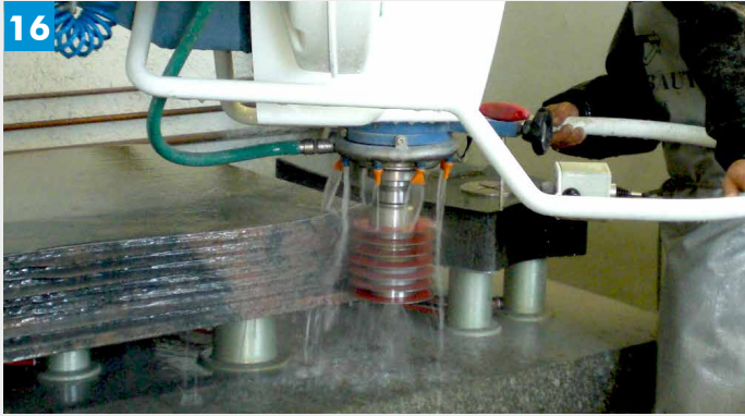
EN Quick shaping with multidisc FR Ebauche rapide au multidisque DE Schnellformgebung mit Trennscheiben Paket ES Desbaste rápido con el multidisco
